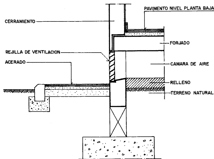
DETALLE DE VENTILACIÓN EN FORJADO DE PLANTA BAJA
